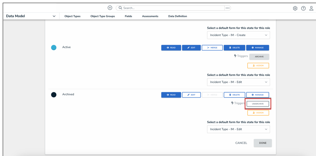
UnarchiveTrigger
