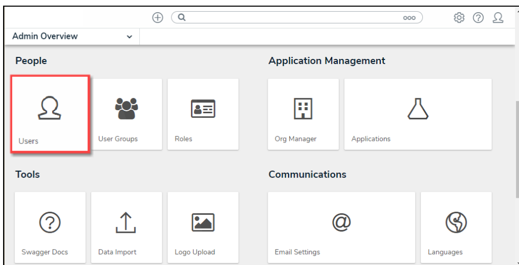
Users Tile
