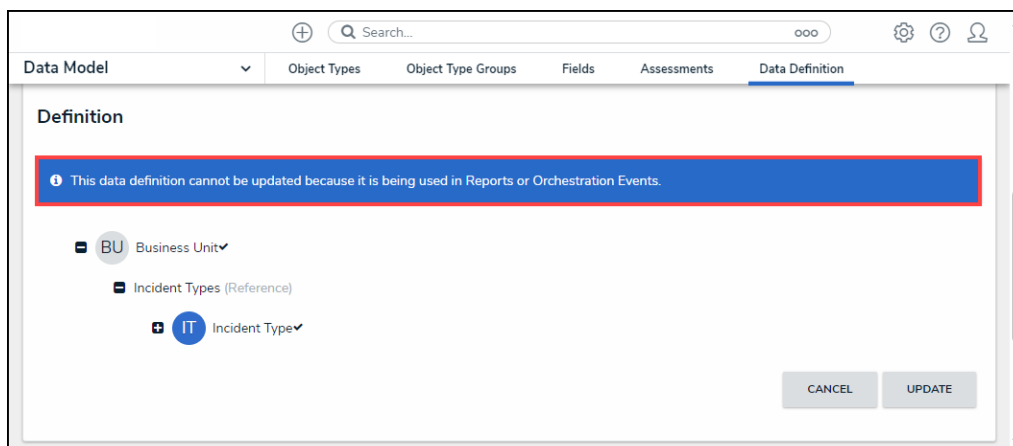
System-Generate Message
